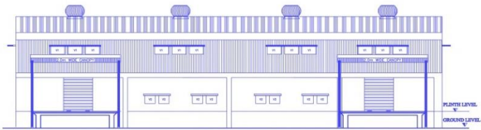
ELEVATION
